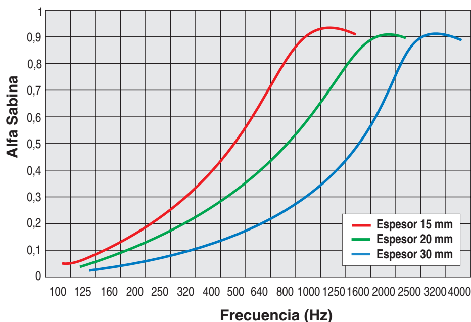
GRÁFICO DE ABSORCIÓN ACÚSTICA Según UNE 74.041-80
