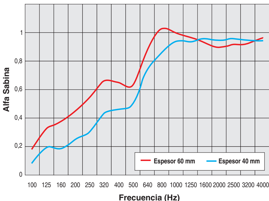
GRÁFICO DE ABSORCIÓN ACÚSTICA Según UNE 74.041-80
