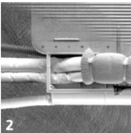
Detalle entrada tubos y cable
