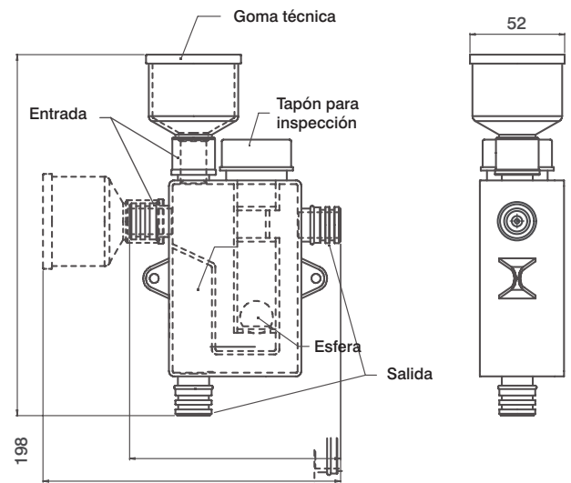
Detalle de la conexión de montaje
