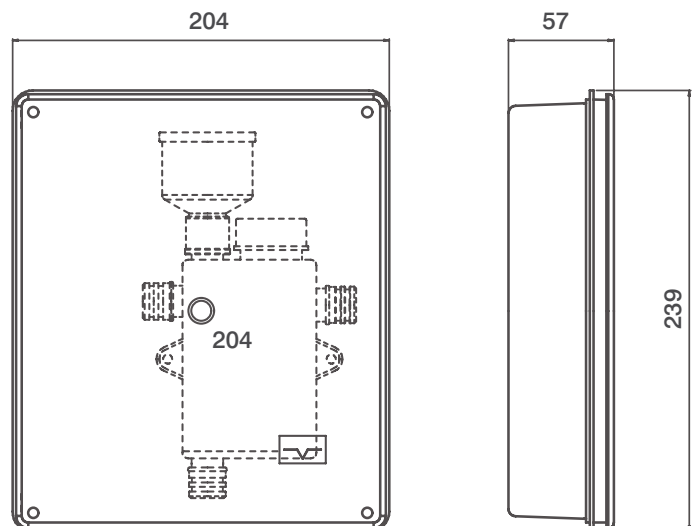
Dimensiones del sifón con caja
