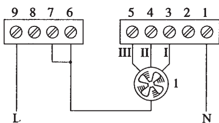
a) Control sobre la velocidad preseleccionada del ventilador.
