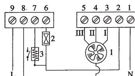
c) Control en invierno sobre el relé de mando de la resistencia y en verano sobre el relé de entrada de agua fría.
