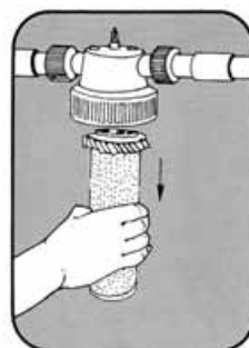
3 Quitar el soporte del filtro.
