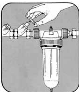
1 Cerrar las válvulas. Abrir las purga.
