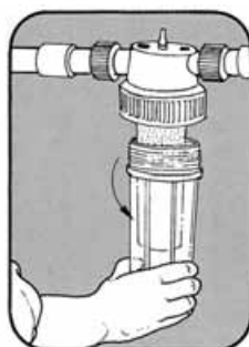
2 Desmontar el vaso del filtro.
