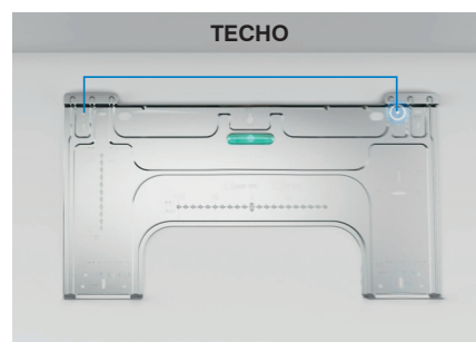
PASO 3: Localizar el punto de fijación en el otro lado con la ayuda del nivel de burbuja
