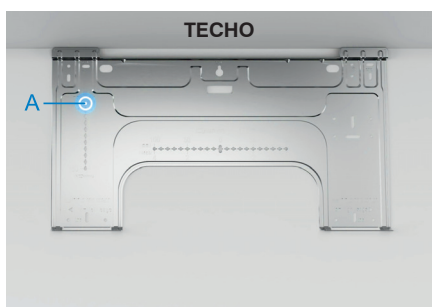
PASO 1: Apoyar la placa contra el techo, marcar el punto A según la altura deseada
