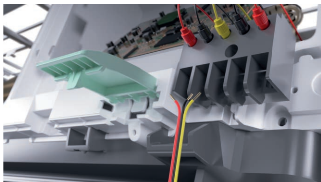
Cuadro eléctrico frontal de fácil acceso, simplemente abriendo el panel frontal. Solo 3 segundos
