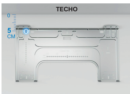
PASO 2: Mover la placa hacia abajo hasta que el agujero de fijación llegue al punto A
