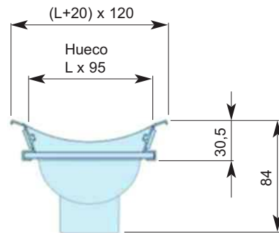
MODELO BIR CON PERFIL Boca inductora regulable con perfil para conductos circulares o cuadrados. L = Longitud del perfil. Cada 100 mm. hay que aumentarle 0,5 mm.
