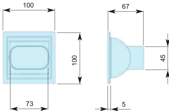
MODELO BIR Boca inductora regulable.
